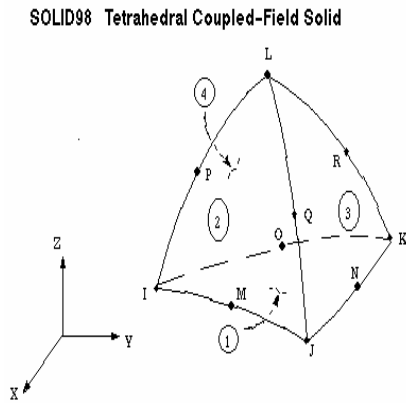
Fig. 2. SOLID98 element
