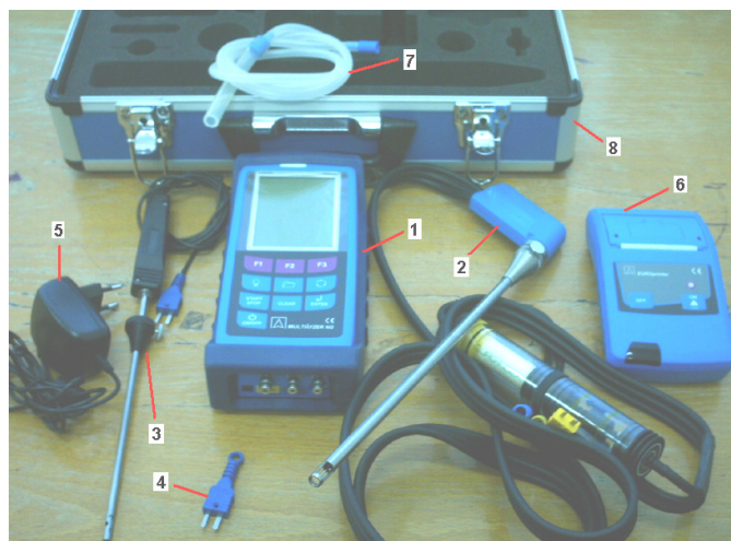
Fig. 3. Kitul de măsurare al analizorului de gaze de ardere Multilyzer N.G 1 – unitatea centrală, 2 – sondă de prelevare,
