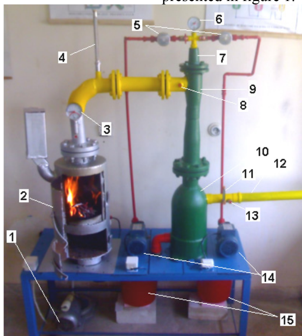
Fig. 1. Instalația pilot folosită la testarea sorbenților
