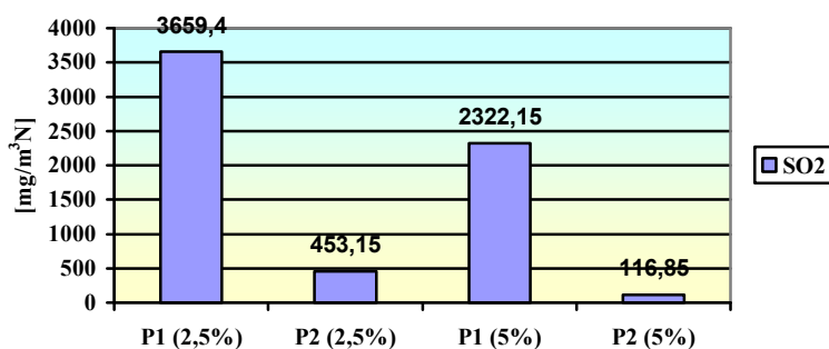
Fig. 4. Rezultate obținute în urma desulfurării gazelor de ardere cu hidroxid de calciu de concentrație 2,5 și 5%
