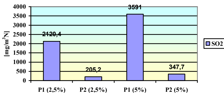
Fig. 5. Rezultate obținute în urma desulfurării gazelor de ardere cu hidroxid de sodiu de concentrație 2,5 și 5%
